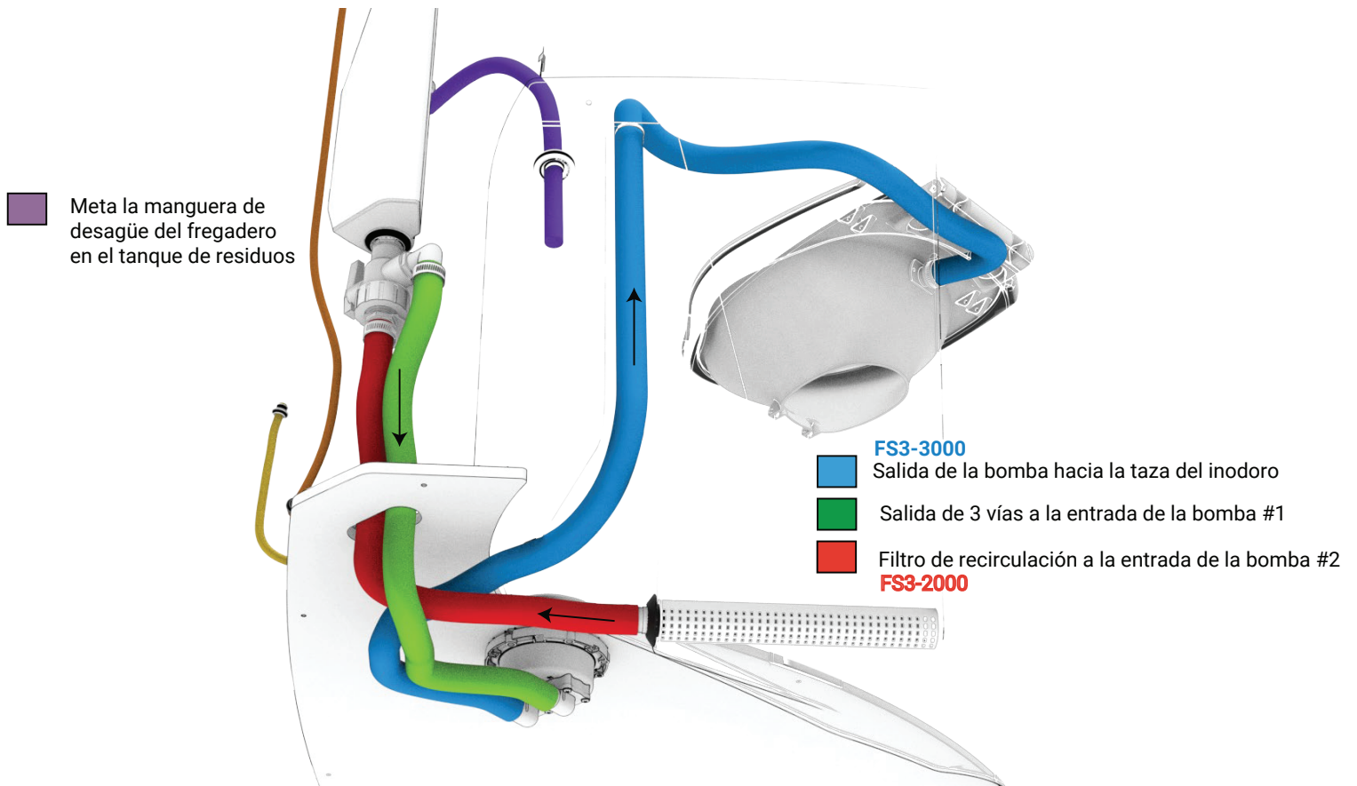
FS3-2000/3000 Conexiones de manguera de descarga con válvula de 3 vías instalada.
